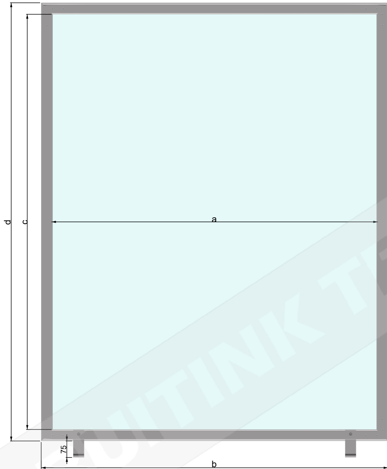
Vooraanzicht [1:10]
